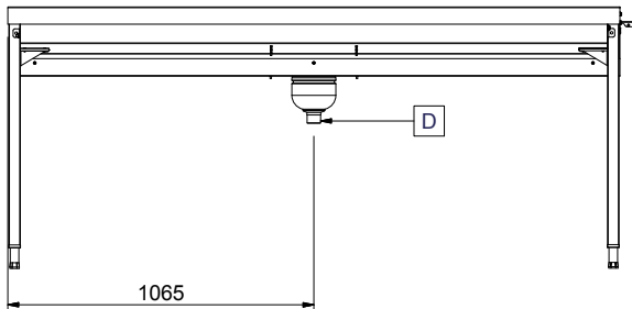
Zij aanzicht
