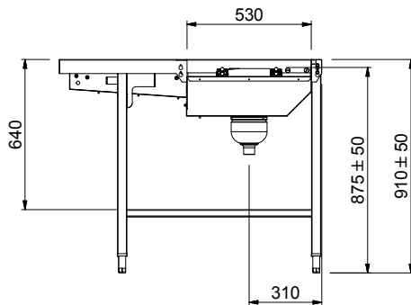
Zij aanzicht
